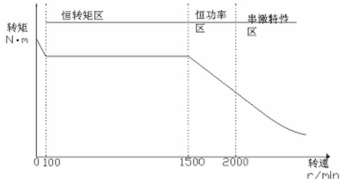
电动机机械特性
